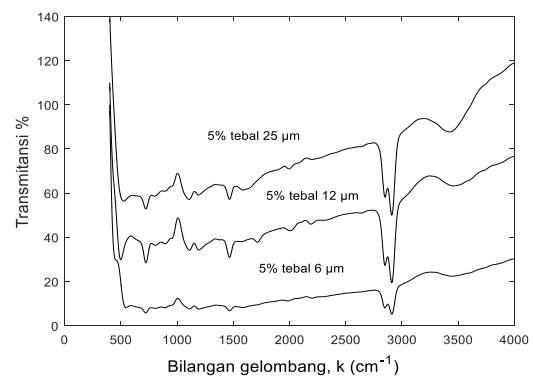
Gambar 1. Spektrum FTIR komposit PE/nanosilika dengan filer 5 %.
