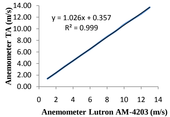
Gambar 7. Grafik hubungan antara anemometer TA rata-rata dengan anemometer Lutron AM-4203
