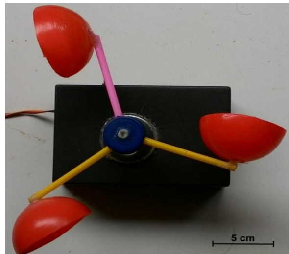
Gambar 2. Perangkat keras kecepatan Angin
