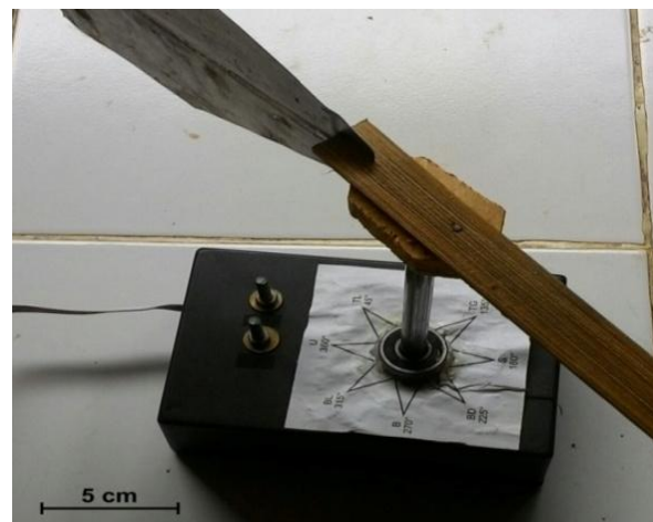
Gambar 3. Perangkat keras arah angin
