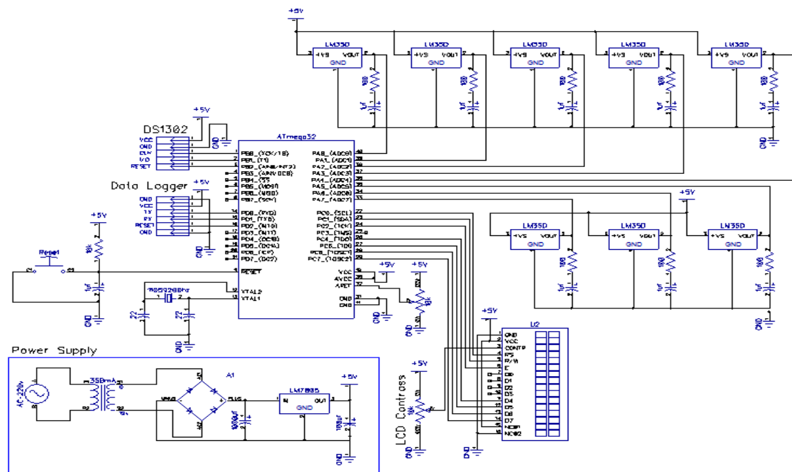
Gambar 3. Rangkaian keseluruhan alat kecepatan aliran fluida
