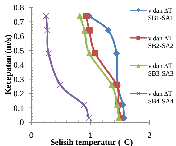
Gambar 5. Grafik selisih temperatur delapan buah sensor LM35DZ dan kecepatan aliran fluida
